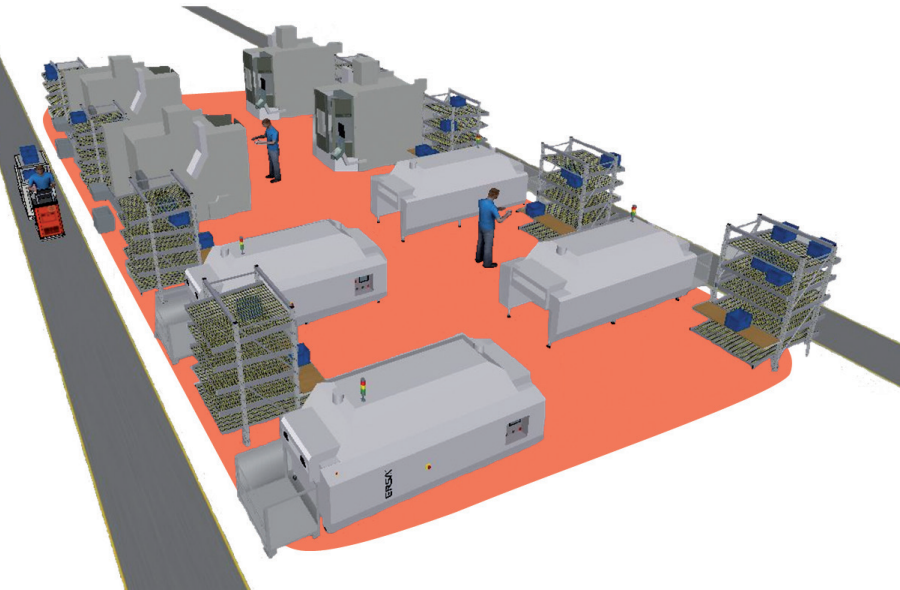
Bild 3: Layout mit Kanban-Regalen und Materialversorgung per Routenzug [12]
