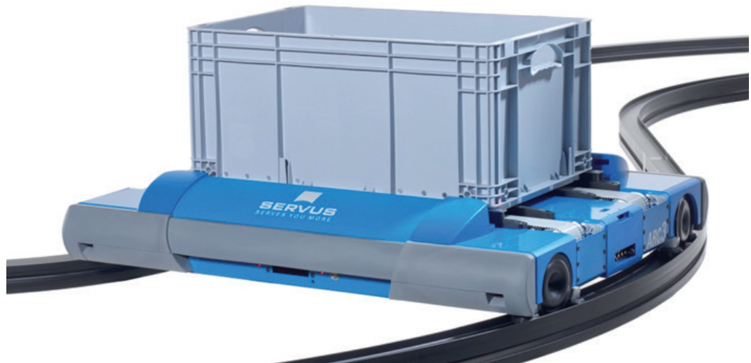
Bild 1: Schematische Darstellung des „Servus ARC 3“ (Autonomous Robotic Carrier)
